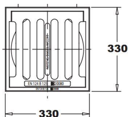
Maatvoering kolkkop bovenaanzicht
